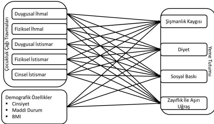
Şekil 1. Hipotetik model
